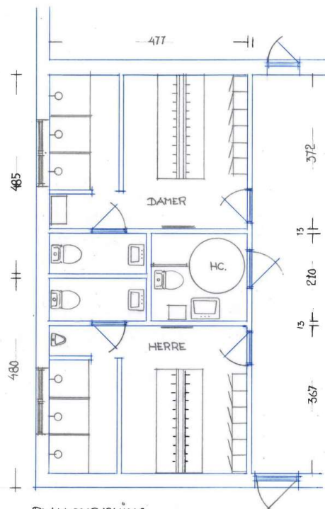
PLAN OMBYGNING HERRE OG DAMETOILETTER + HC-TOILET MÅL 1:50 DATO 23-10-2021 / VW3
