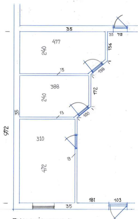
PLAN EKST. FORHOLD HERRE OG DAMETOILETTER + GREENKEAPERRUM MÅL 1:50 DATO 23-10-2021 / VW3
